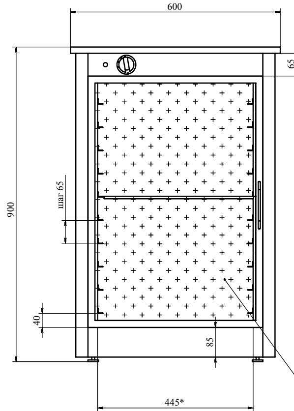
Вид спереди (1:10)
