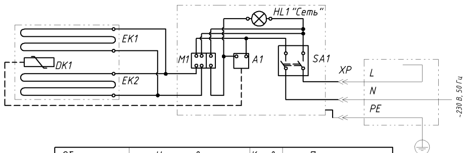
Мармит вторых блюд СХЕМА ЭЛЕКТРИЧЕСКАЯ ПРИНЦИПАЛЬНАЯ
